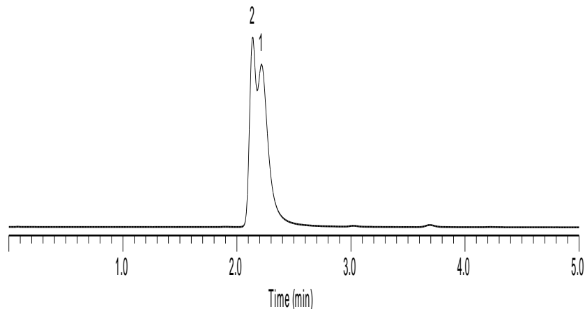
*SMT C18
