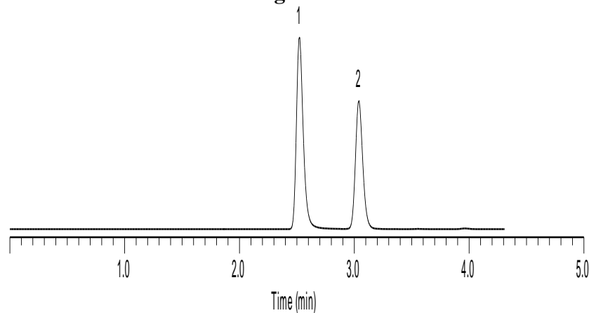
*Agilent TC-C18
