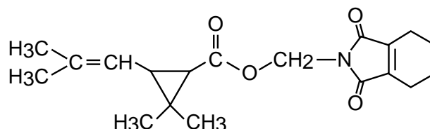
phthalthrin (tetramethrin)
